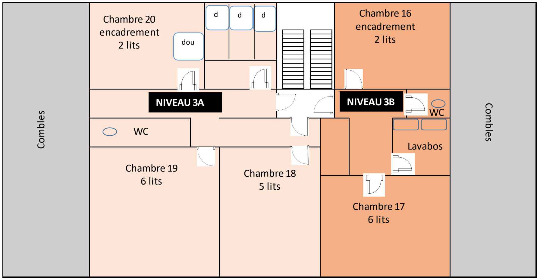
Niveau 3 (21 lits)
